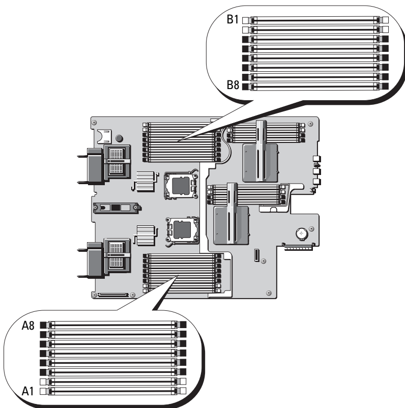
図 3-8. メモリの位置 - PowerEdge M805
